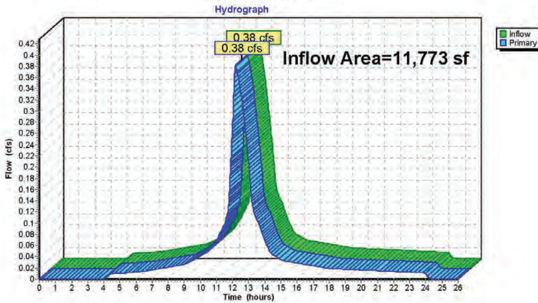
Link 3L: storm sewer
